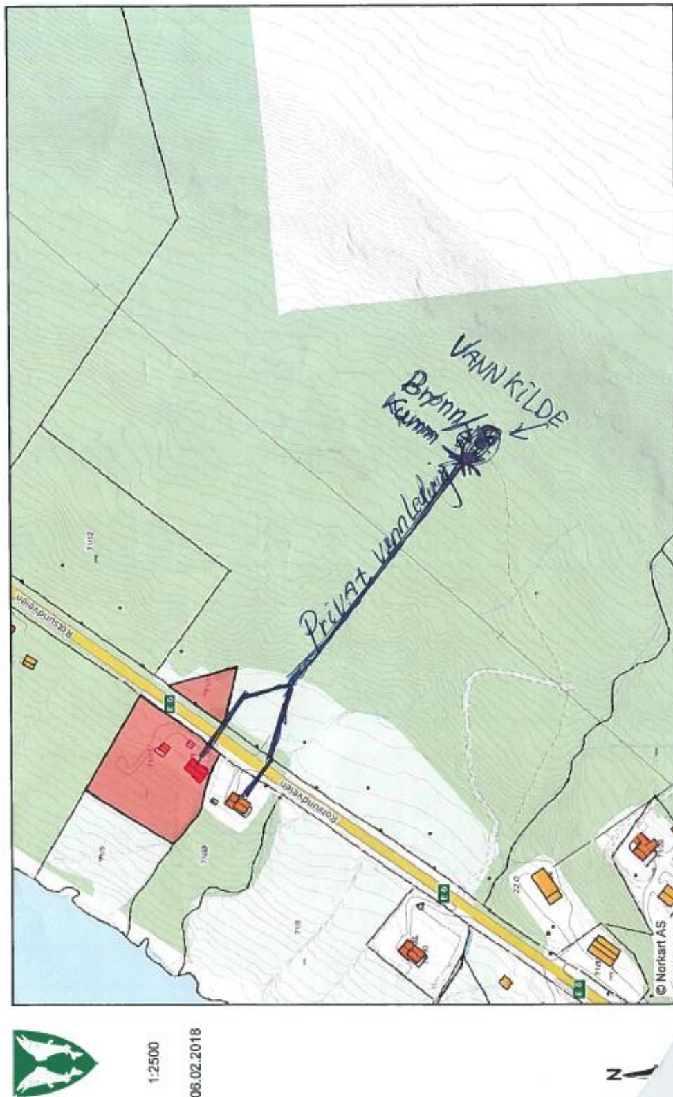
Figur 12 Kartskisse privat vannledning på eiendommen gbnr. 71/6
