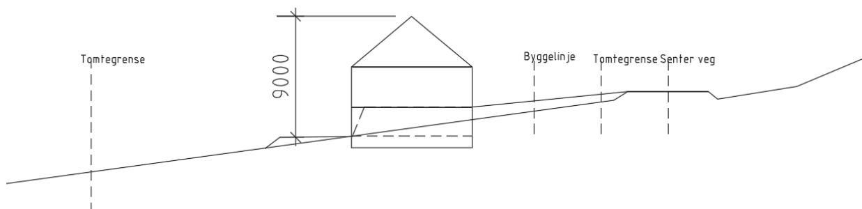
Figur 14 Illustrasjon mønehøyde
