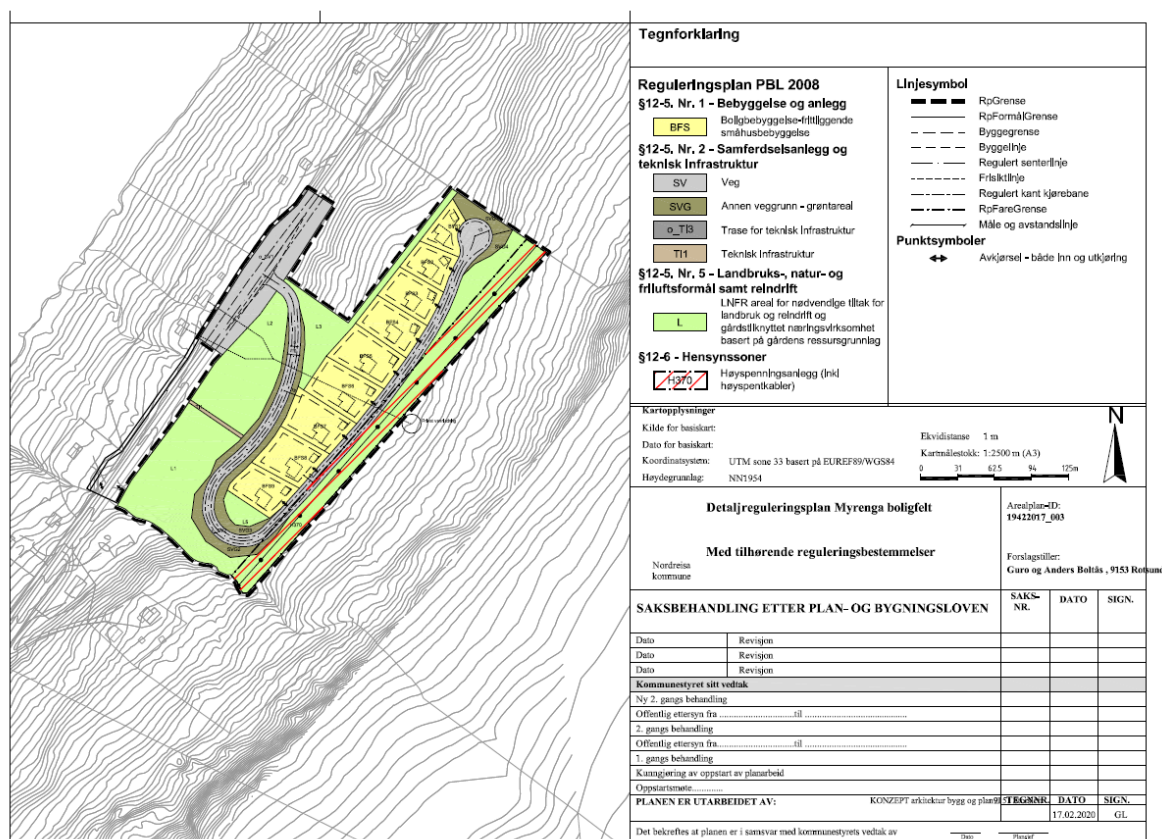
Figur 13 Plankart Detaljregulering Myrenga boligfelt
