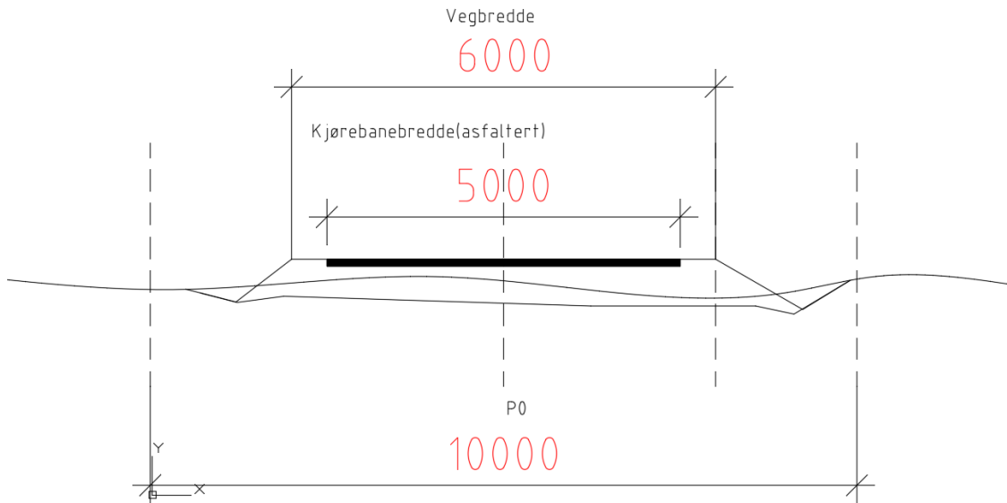
Figur 15 Tverrsnitt for veg o-Sv2 ved avkjøring fra E6
