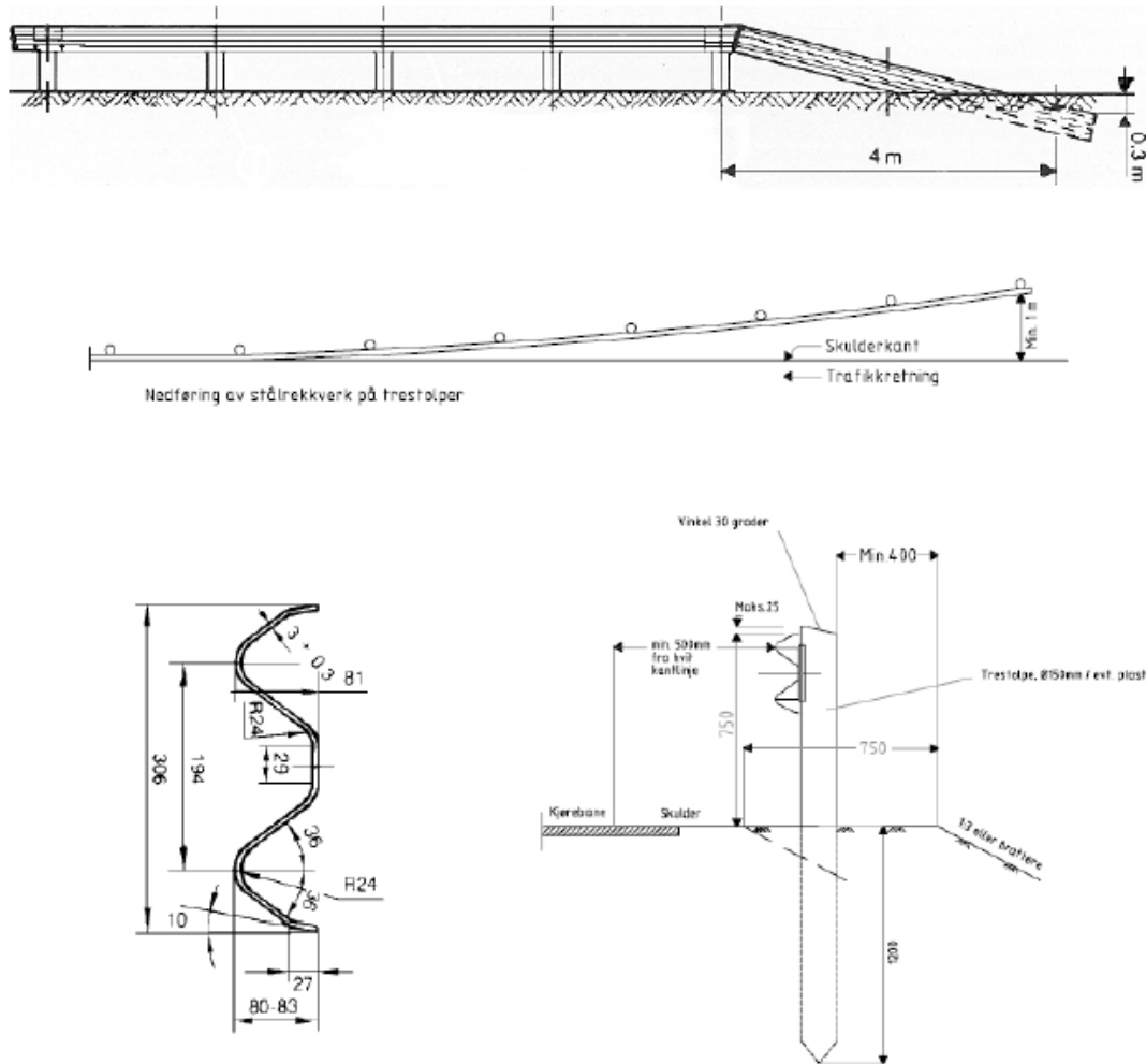
Figur 16 Illustrasjon på autovern
